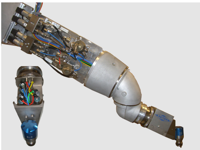
Roboter-Prozessarm
