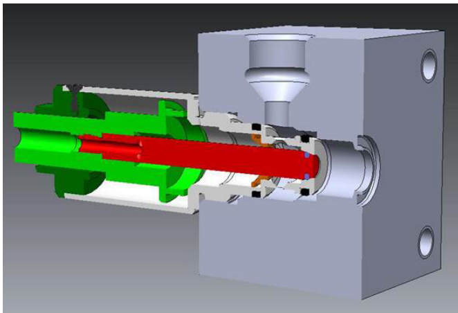
Standardventil im Farbwechselblock
