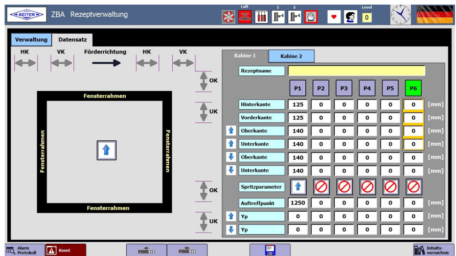
Vergrößerung und Verkleinerung der Werkstücke. Individuelle Einstellung der Pistolenschaltpunkte programmierbar.
